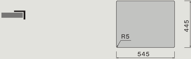
Installation à fleur Schéma d'encastrement
