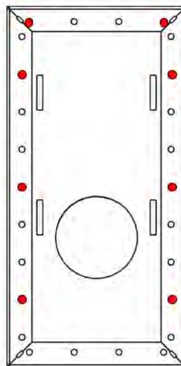
Figure n°10 - Position des vis
