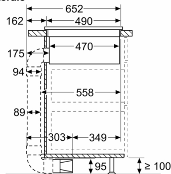
Mesures en mm Vue latérale
