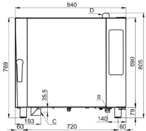
Vue face
