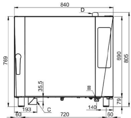
Vue face
